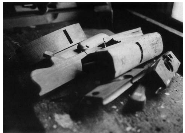
Bild9. Några av Mjöbäckswerkstadens många bevarade specialverktyg, här profilhyvlar. Foto: Hallands läns museer, B. Petersen 1991.
